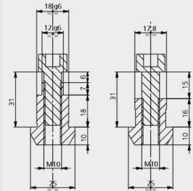
► T-SLOT 18 46204105
