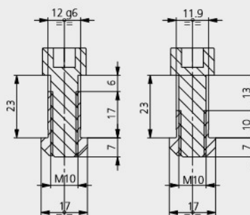
► T-SLOT 12 46204103
