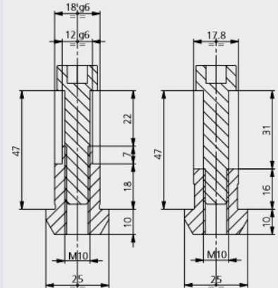
► T-SLOT 18 46204102
