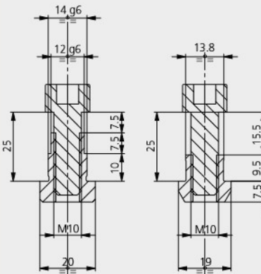
► T-SLOT 14 46204104
