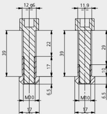
► T-SLOT 12 46204100
