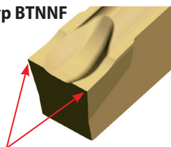
Kein Eckenradius Sharp edge without radius
